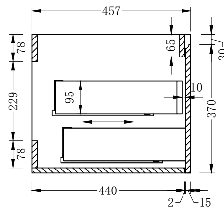
SEZIONE A-A
