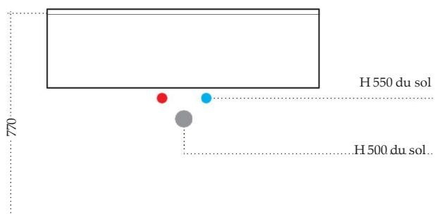
BASES 60 - 80 avec plan de toilette
