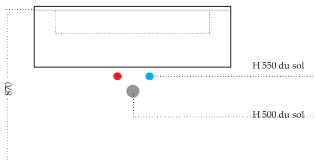
BASES 60 - 80 avec plan vasque
