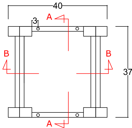
TOP VIEW T. Atas
