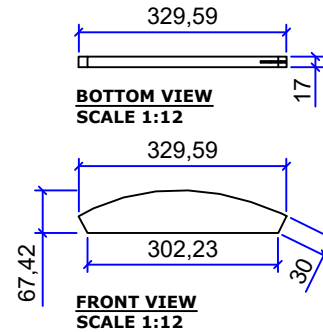
FRAME TEGAK 2 Qty : 1 pcs
