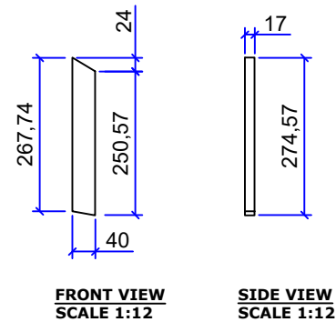
FRAME TEGAK 2 Qty : 1 pcs
