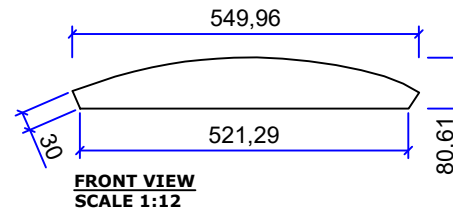
FRAME MIRROR 4 Qty : 1 pcs
