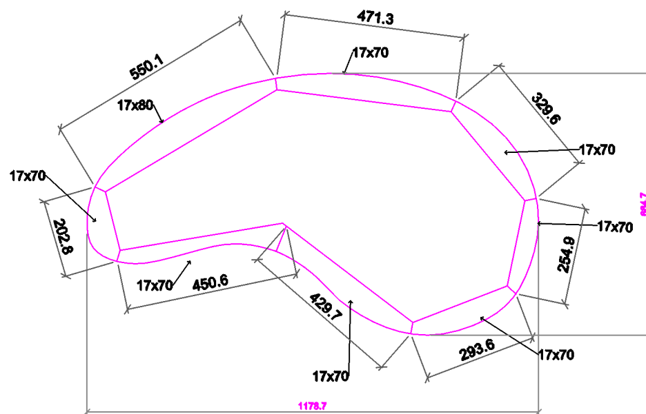
pola potong kayu
