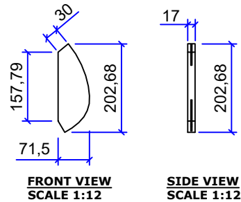
FRAME MIRROR 5 Qty : 1 pcs
