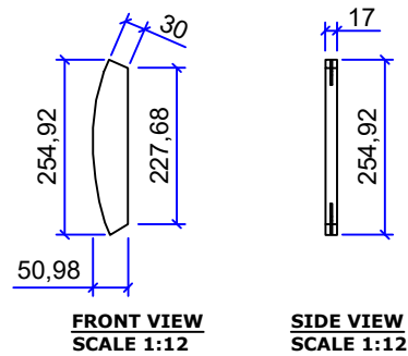
FRAME TEGAK 1 Qty : 1 pcs
