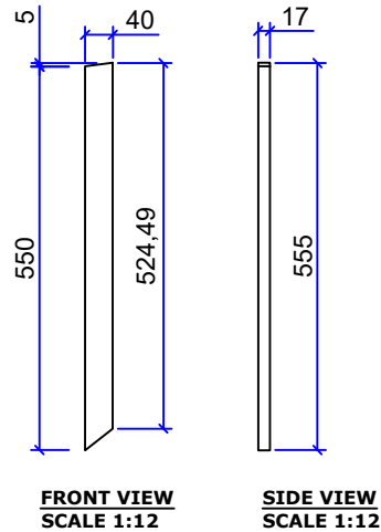
FRAME TEGAK 1 Qty : 1 pcs
