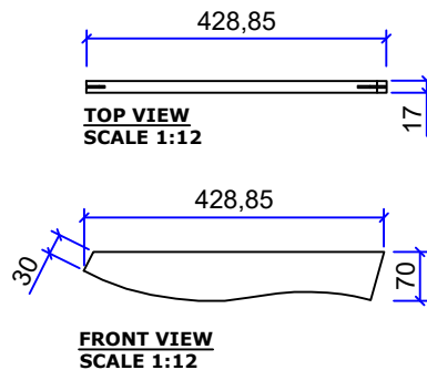
FRAME MIRROR 5 Qty : 1 pcs
