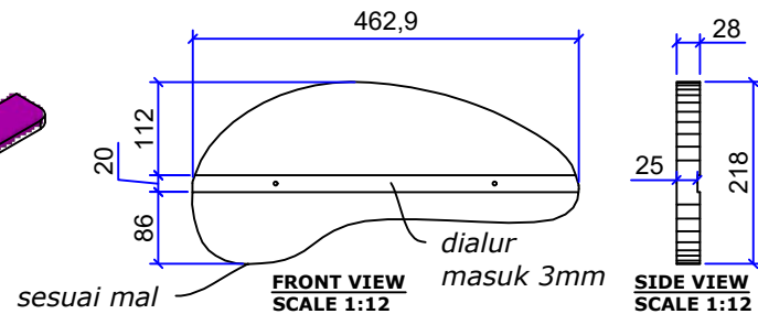
SHELF Qty : 1 pcs
