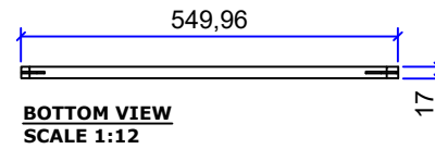
FRAME MIRROR 2 Qty : 1 pcs
