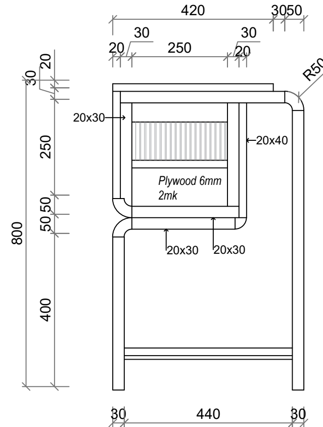
T. BELAKANG SCALE 1:10
