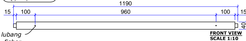
3.1 SUNDUK ATAS Qty : 1 pcs
