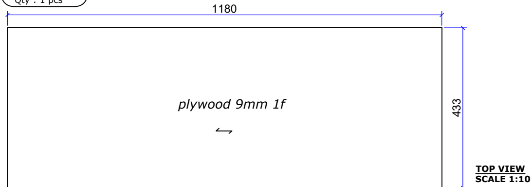
4.1 DASARAN Qty : 1 pcs
