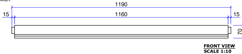
3.2 SUNDUK BAWAH Qty : 1 pcs
