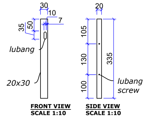
2.3 DUDUKAN KH 150 Qty : 2 pcs
