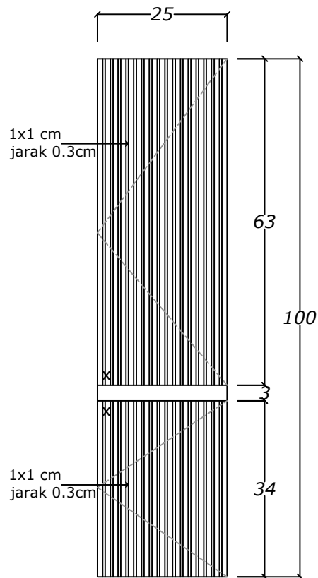
Tampak Depan
