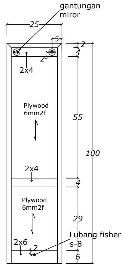
Tampak Belakang
