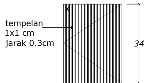
PINTU T.DEPAN
