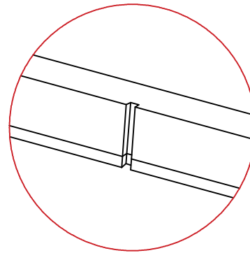
Detail Alur Kabel Lebar 8mm dalam 5 mm
