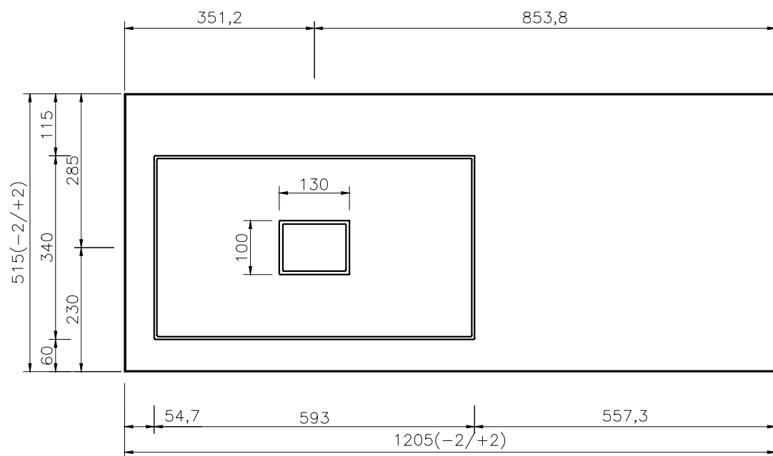
SCALA 1:10
