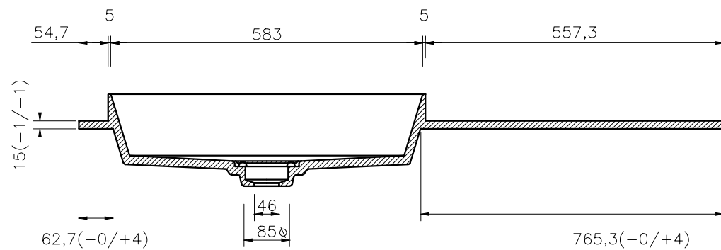
SEZIONE A-A SCALA 1:10
